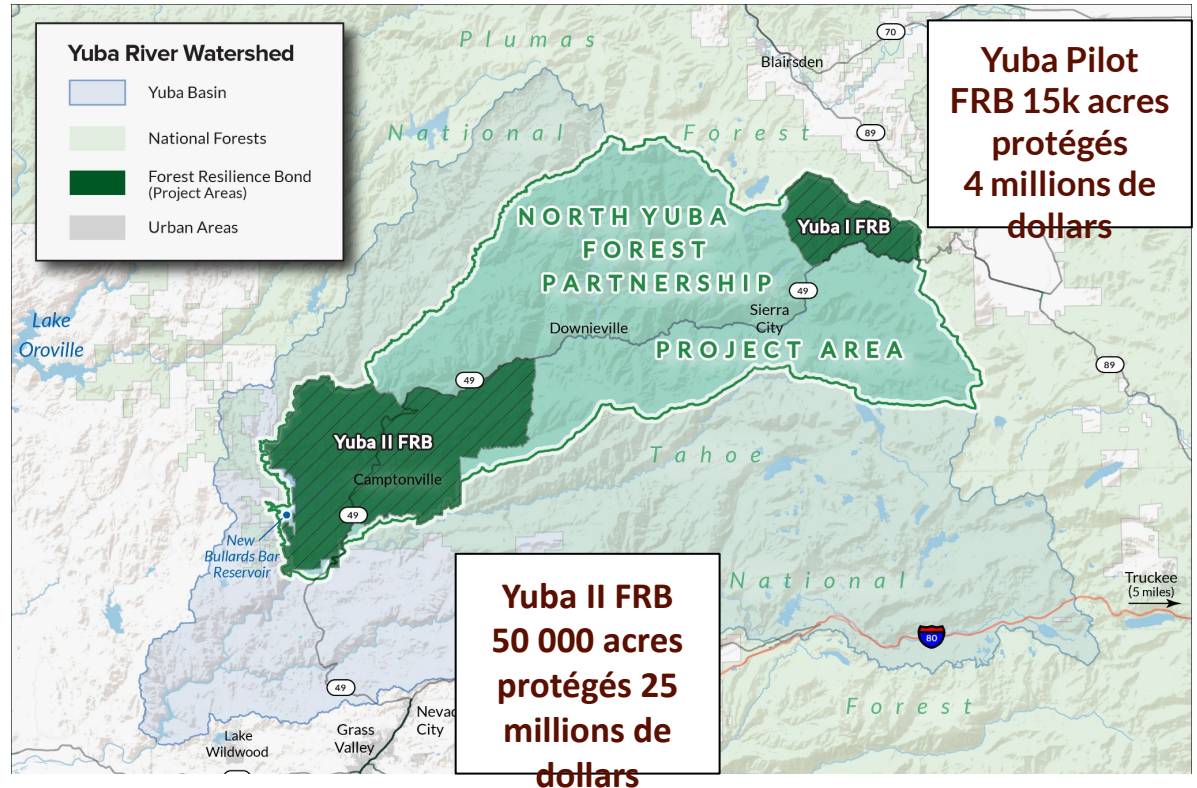
Bassin versant de la rivière Yuba Nord, Tahoe NF, Californie
